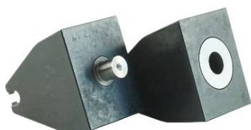
Lochstanzadapter mit montierten Einsätzen
